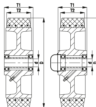
golyóscsapágy
