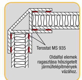
Terostat MS 935
